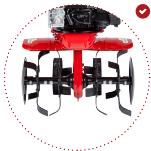
Fresa 40 cm, Ø 26 cm
